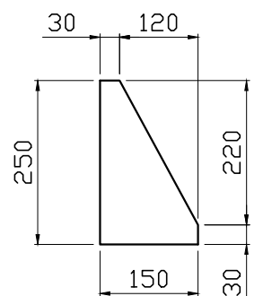
PEÇA B CHAPA #1/4" QUANTIDADE : 08 PÇS
