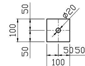
PEÇA 03 CHAPA # 3/8" QUANTIDADE = 08 PÇS.
