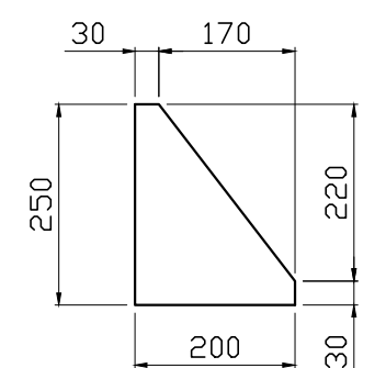
PEÇA A CHAPA #3/8" QUANTIDADE : 04 PÇS
