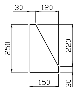
PEÇA C CHAPA #3/8" QUANTIDADE : 04 PÇS
